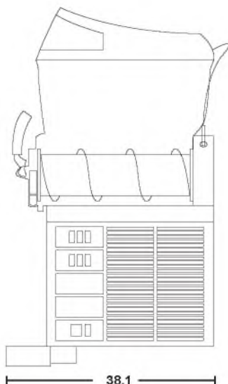
Vista Lateral
